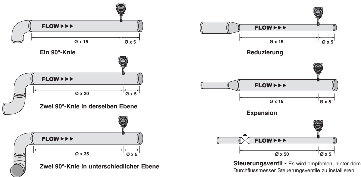
Abbildung C – Installation der Sonden
