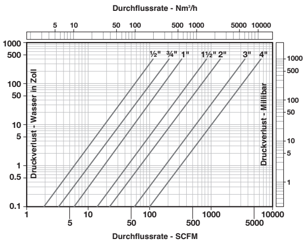
Druckverlust
