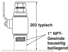
1" NPT-Kugelhahn aus Edelstahl 1.4401 (316 SST) mit Rohrverschraubung (TFE-Klemmringe) Bestellnummer: 089-5218-001
