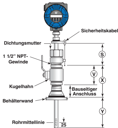
Modell RPA-E402-XXX
