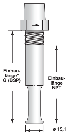
TMR mit Gewindeanschluss
