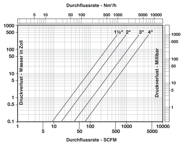
Druckverlust mit Strömungsgleichrichter
