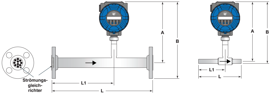
Messstrecke mit Flansch
