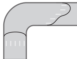
Abbildung B Strömungsprofil entsprechend Einzelknie
