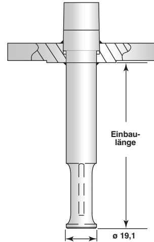
TMR mit Flanschanschluss
